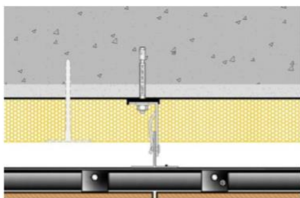
SEZIONE ORIZZONTALE
